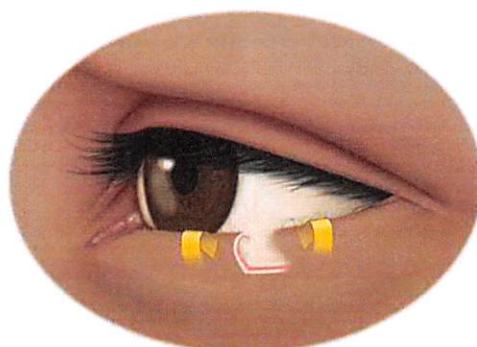
Entropion
