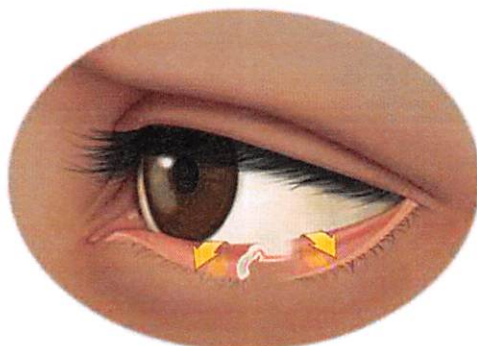
Ectropion
